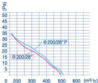
YZF6-13 60Hz Air Flow 空气量
