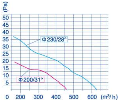
YZF10-20 50Hz Air Flow 空气量
