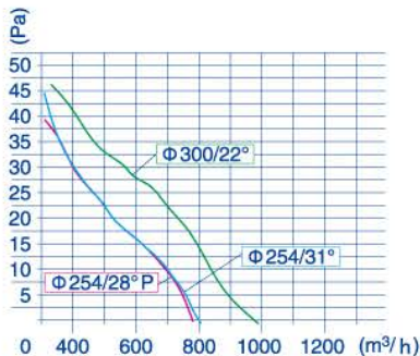
YZF18-30 50Hz Air Flow 空气量
